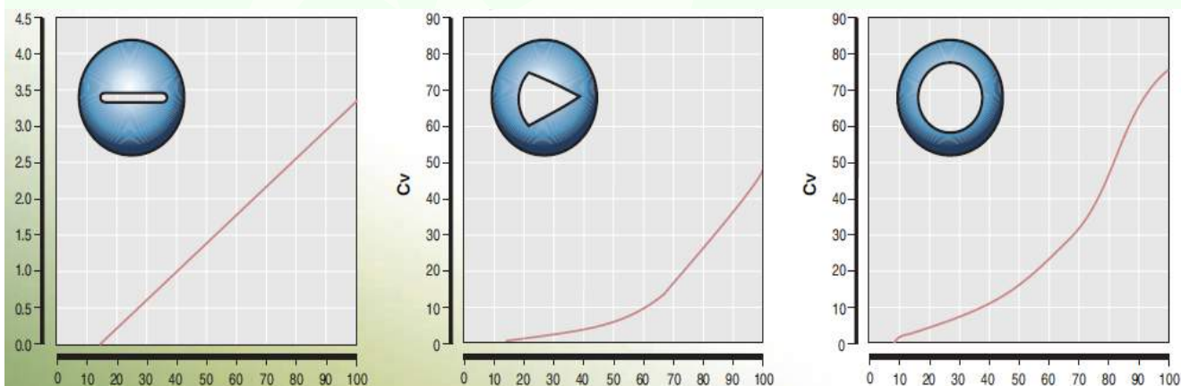
V-Port
